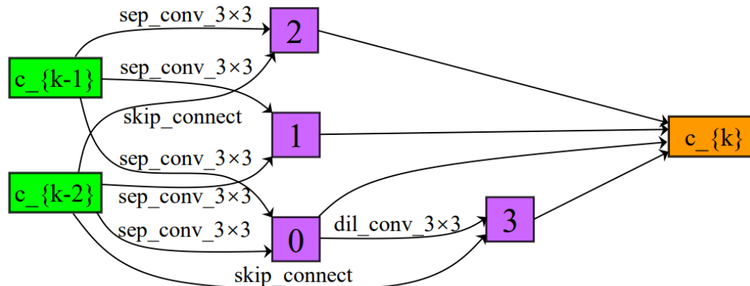
(d) DARTS_V2, CIFAR10 Test Err. 2.83%
