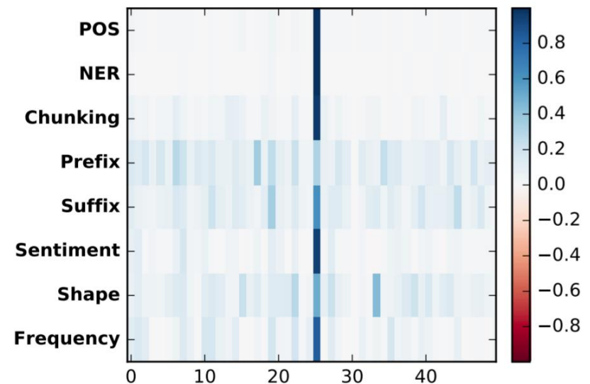
(d) GloVe, no dropout; 31rd dimension removed.
