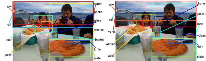
SG-obj
