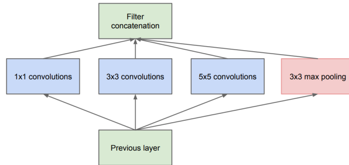
Inception module
