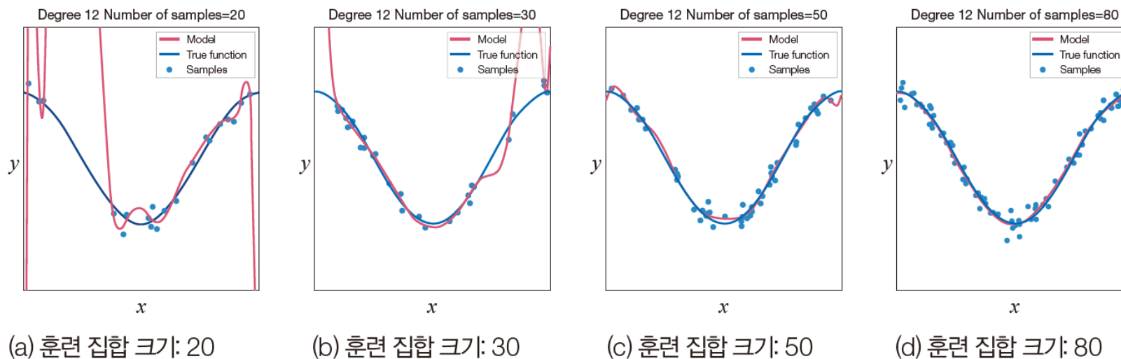
그림 5-14 데이터 양을 늘려 과잉 적합을 해소
