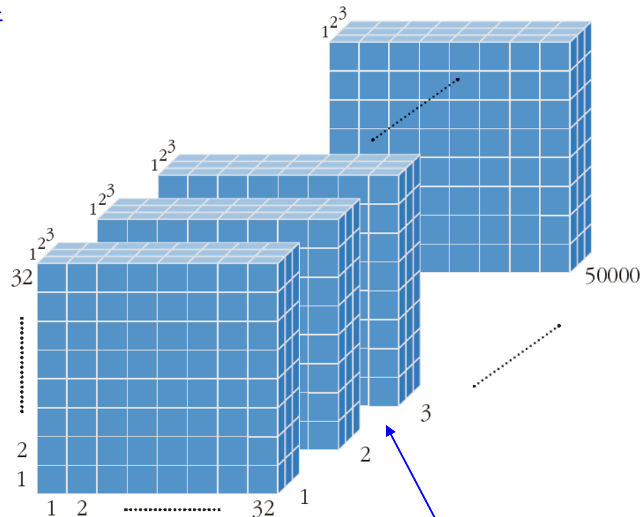
(b) CIFAR-10의 x_train 텐서
