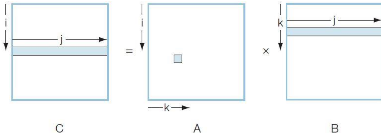
그림 11-6 A의 i 번째 행과 B의 j 번째 열을 곱한 C[i, j]
