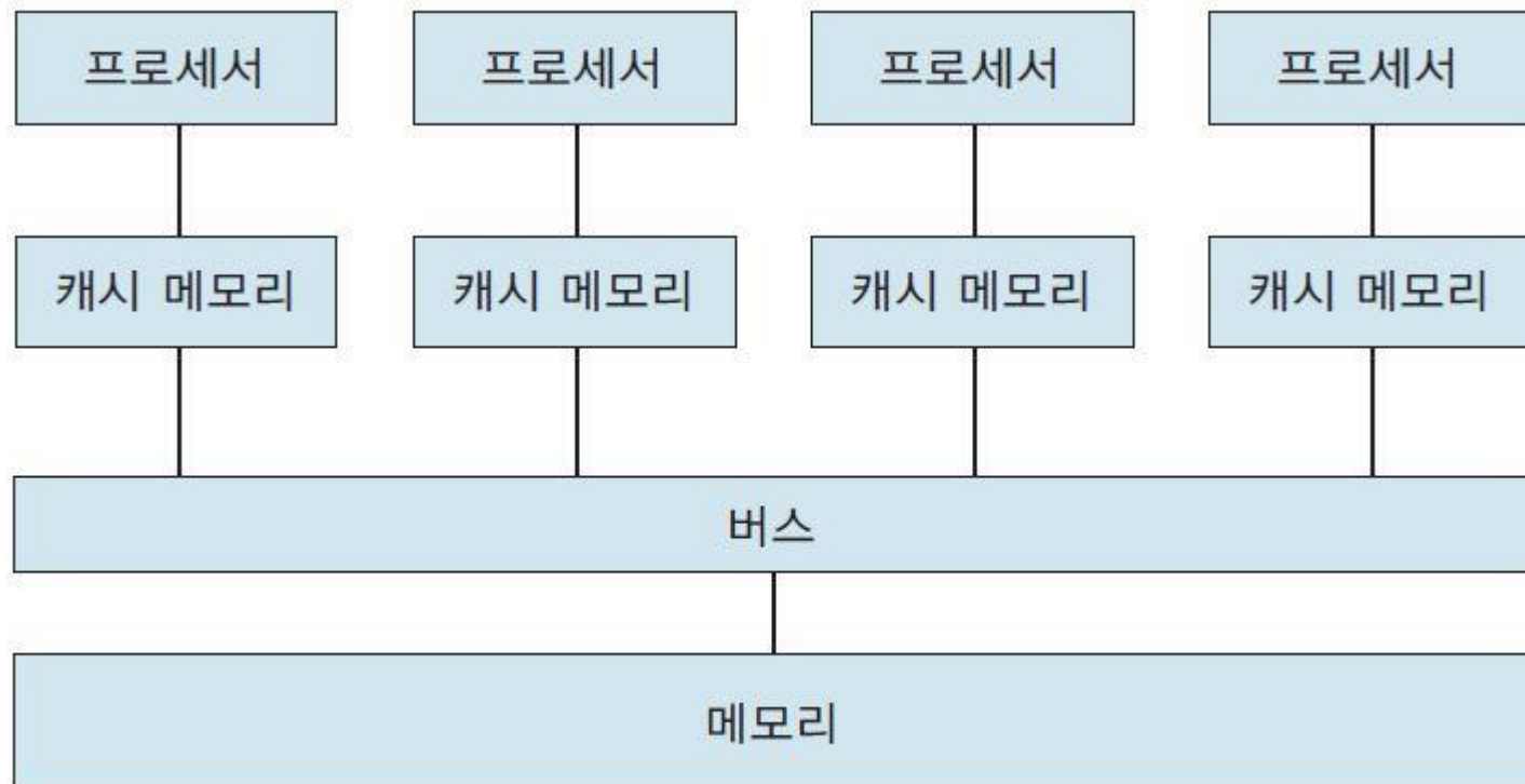
그림 11-1 대칭적 다중 프로세서의 구조
