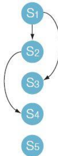
그림 11-11 출력 종속과 반종속이 제거된 자료 종속 그래프
