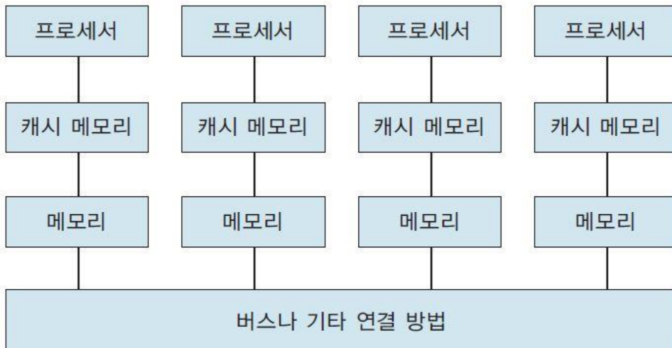
그림 11-2 분산 메모리 시스템의 구조
