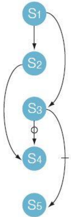
그림 11-9 자료 종속 그래프
