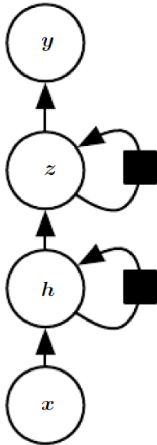
Hierarchical
