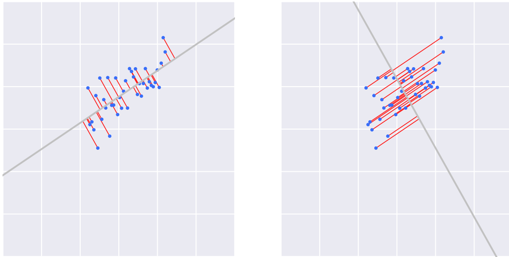
PCA example
