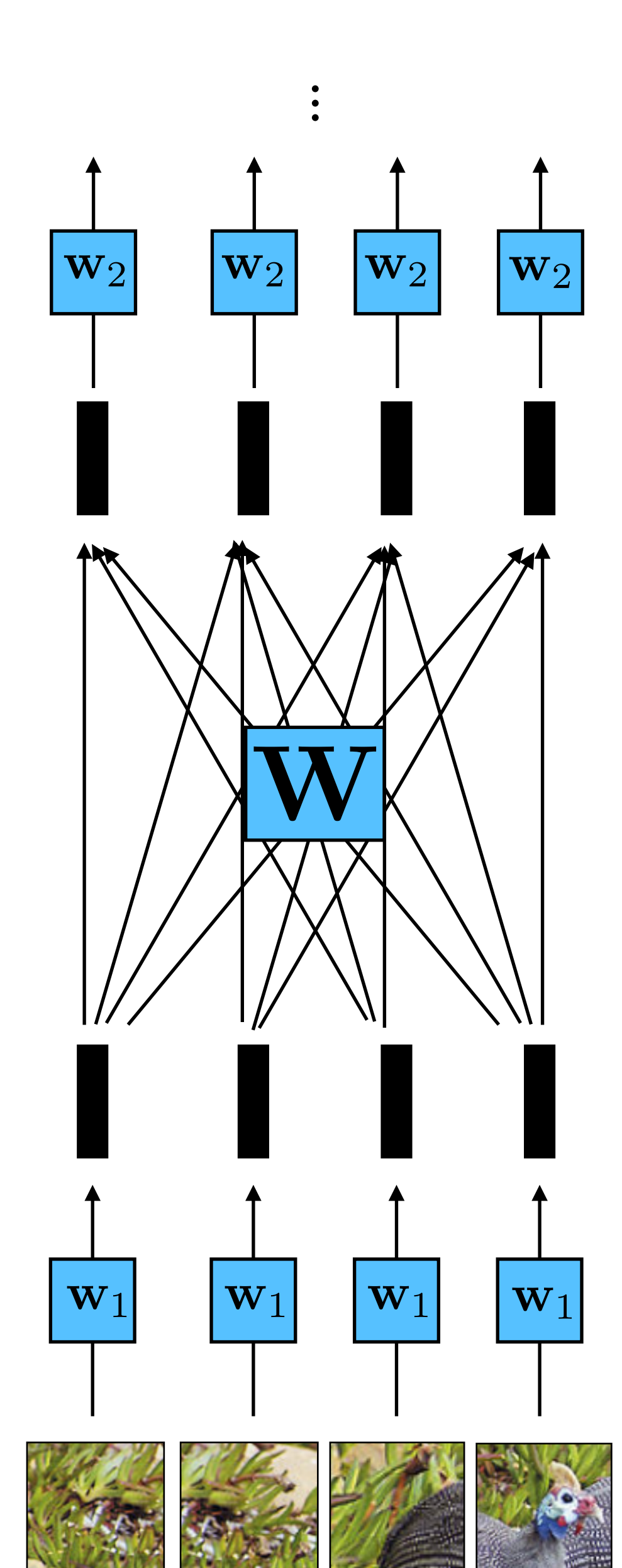
fc layer
